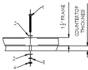
BOLT
